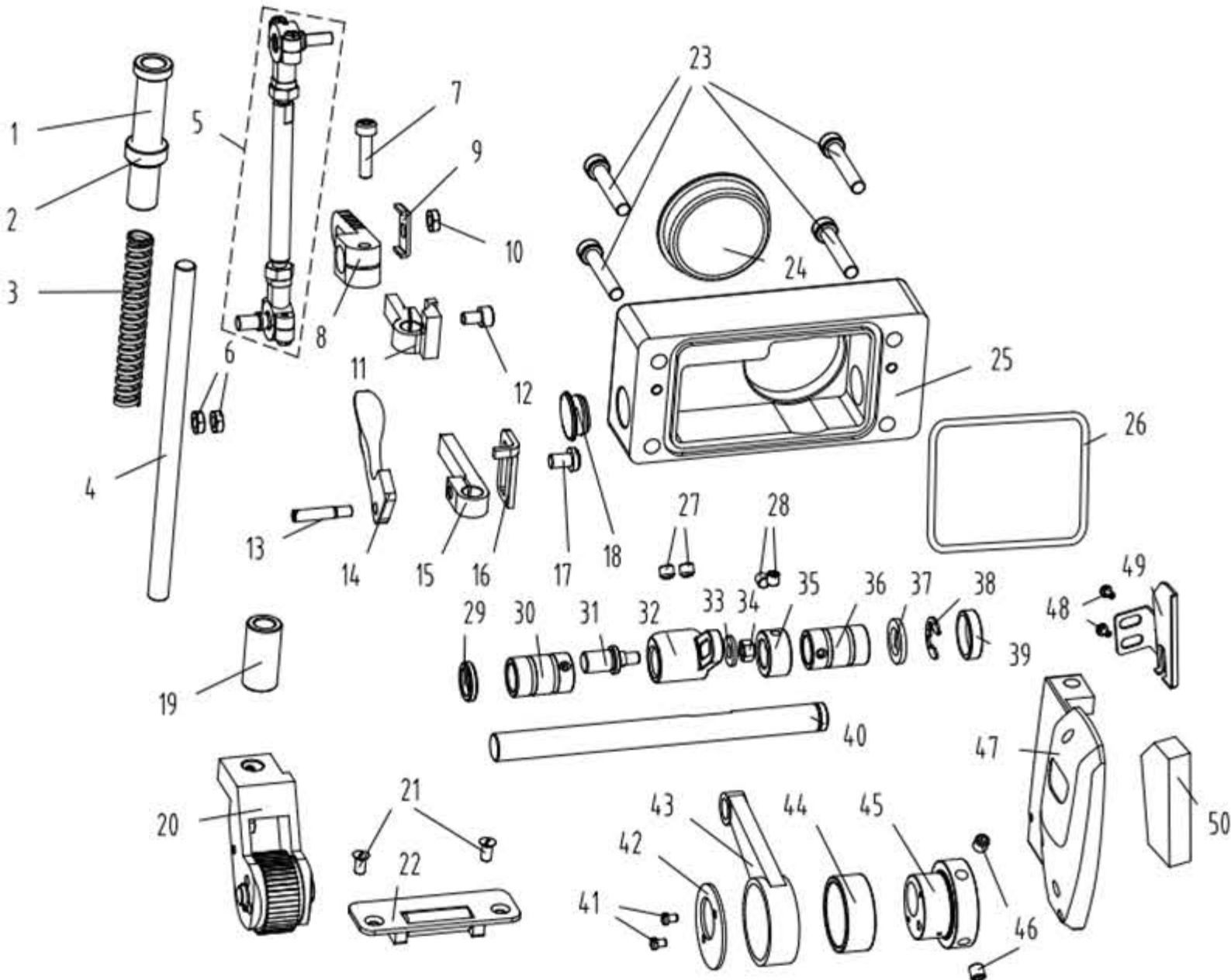
11. 后拖轮装置/ Puller device mechanism
